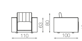
POLTRONA / ARMCHAIR
